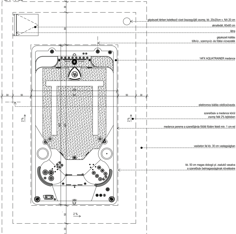
ALAPRAJZ
