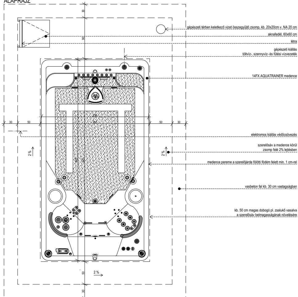
ALAPRAJZ
