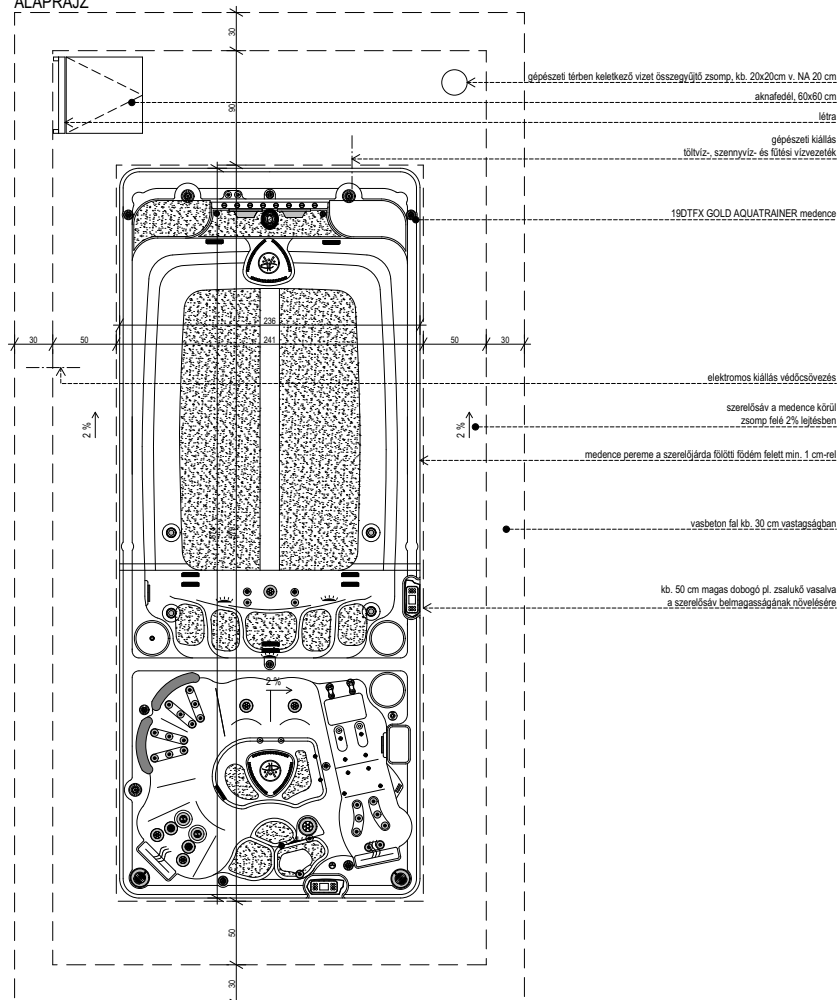
ALAPRAJZ
